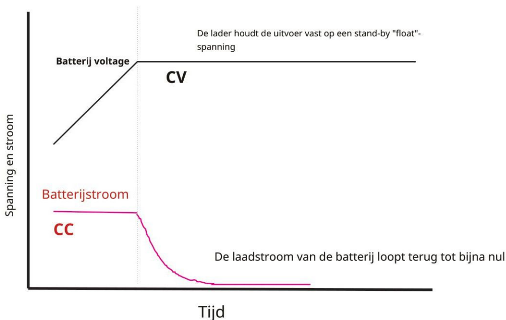
Accuspanning en -stroom tijdens het opladen
